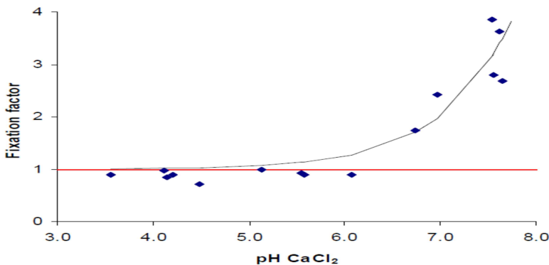
그림 4-7. 토양에서 니켈의 노후화 관련 고정계수와 pH 간의 상관관계
