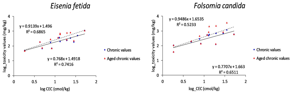
그림 4-8. 토양에서의 만성독성과 양이온교환용량 간의 단일 선형 회귀
