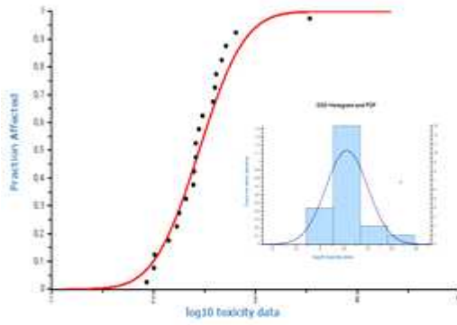
그림 4-9. 니켈에 대한 육상환경 중 민감도 분포
