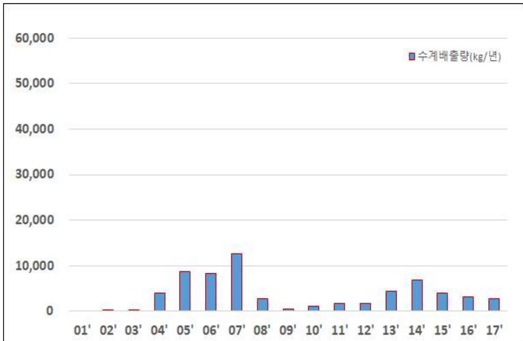
그림 2-4. 니켈 및 그 화합물의 연도별 국내 수계배출량 현황
